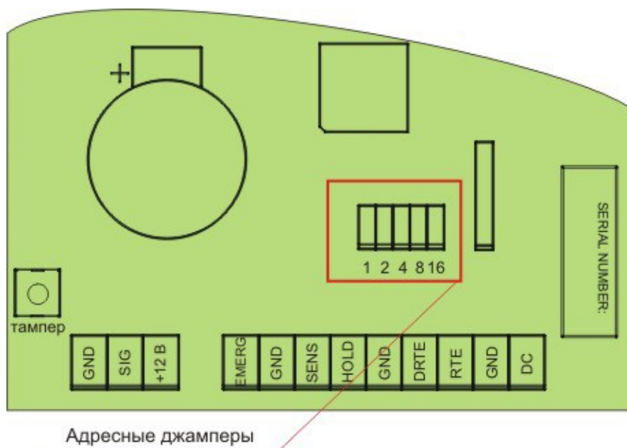
Рисунок 20. Адресные переключики
