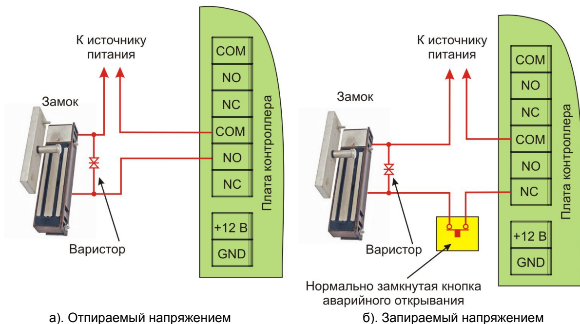
Рисунок 6. Подключение замков к контроллеру
