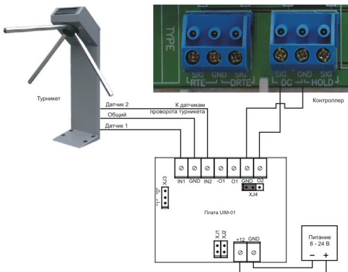
Рисунок 3. Подключение турникета с двумя датчиками проворота.
