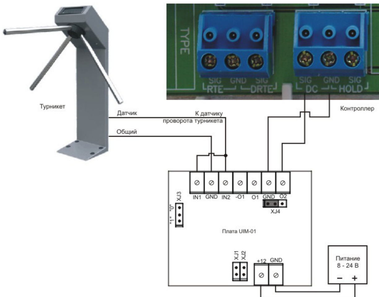
Рисунок 2. Подключение турникета с одним датчиком проворота.
