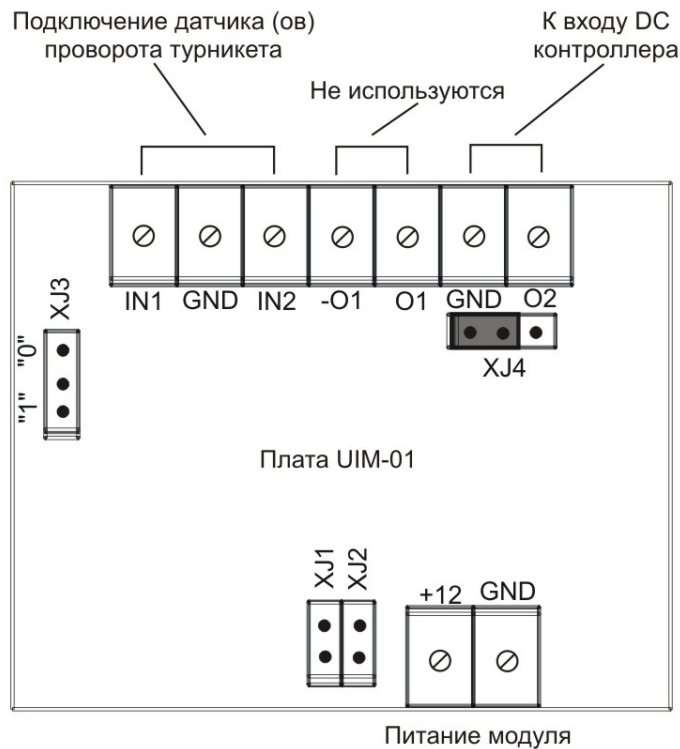
Рисунок 1. Плата модуля сопряжения UIM-01.
